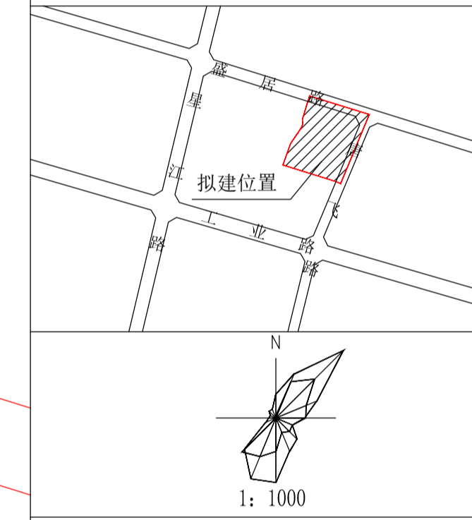
总平面图
